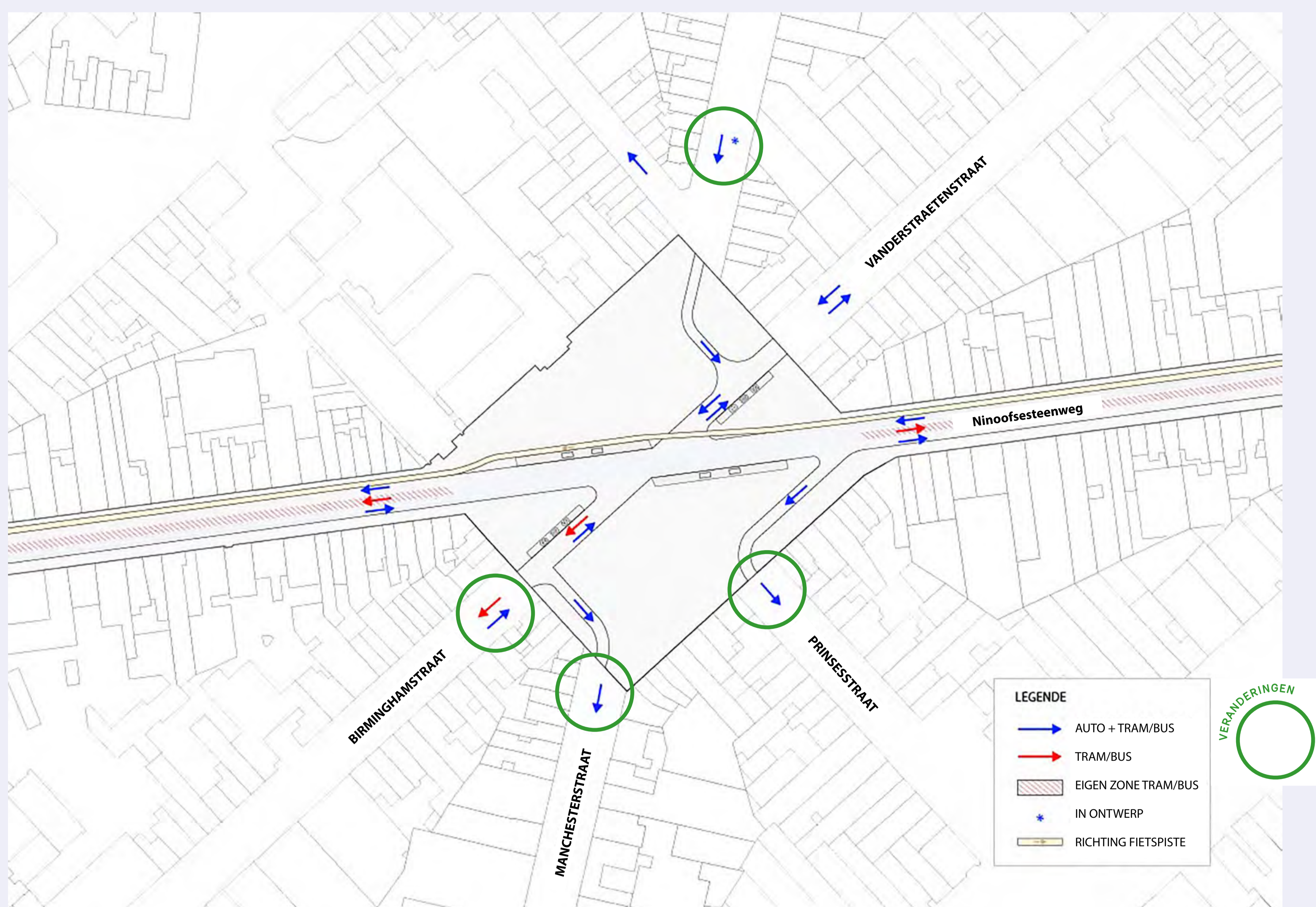
Circulatieplan: ontwerpvoorstel 1
