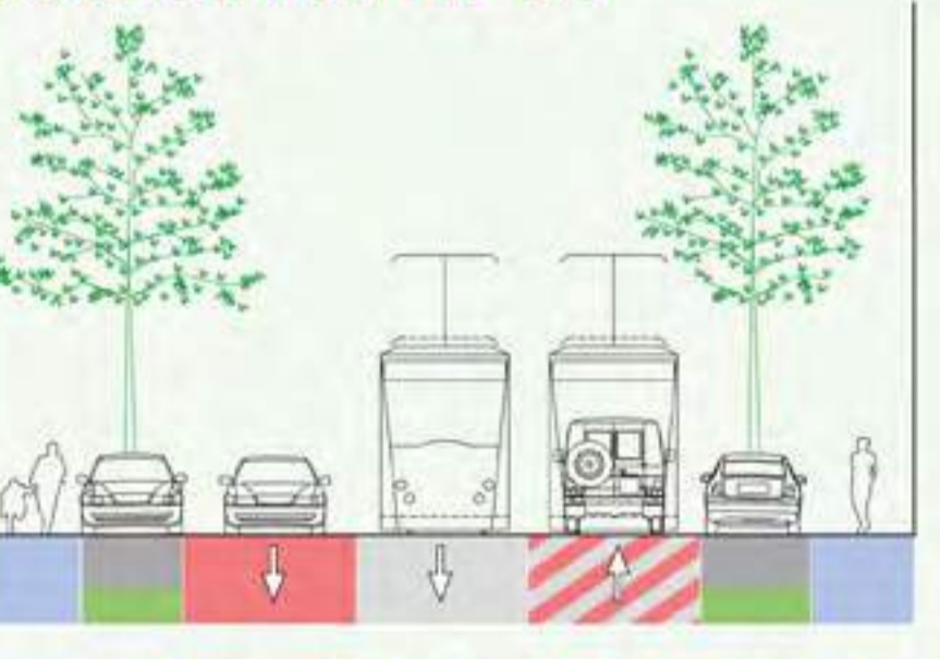
BESTAANDE SITUATIE
