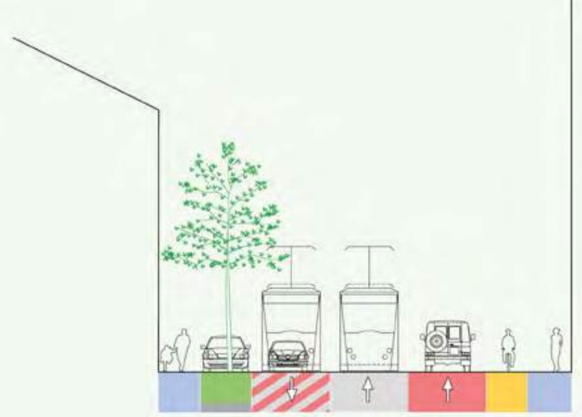
TOEKOMSTIGE SITUATIE
