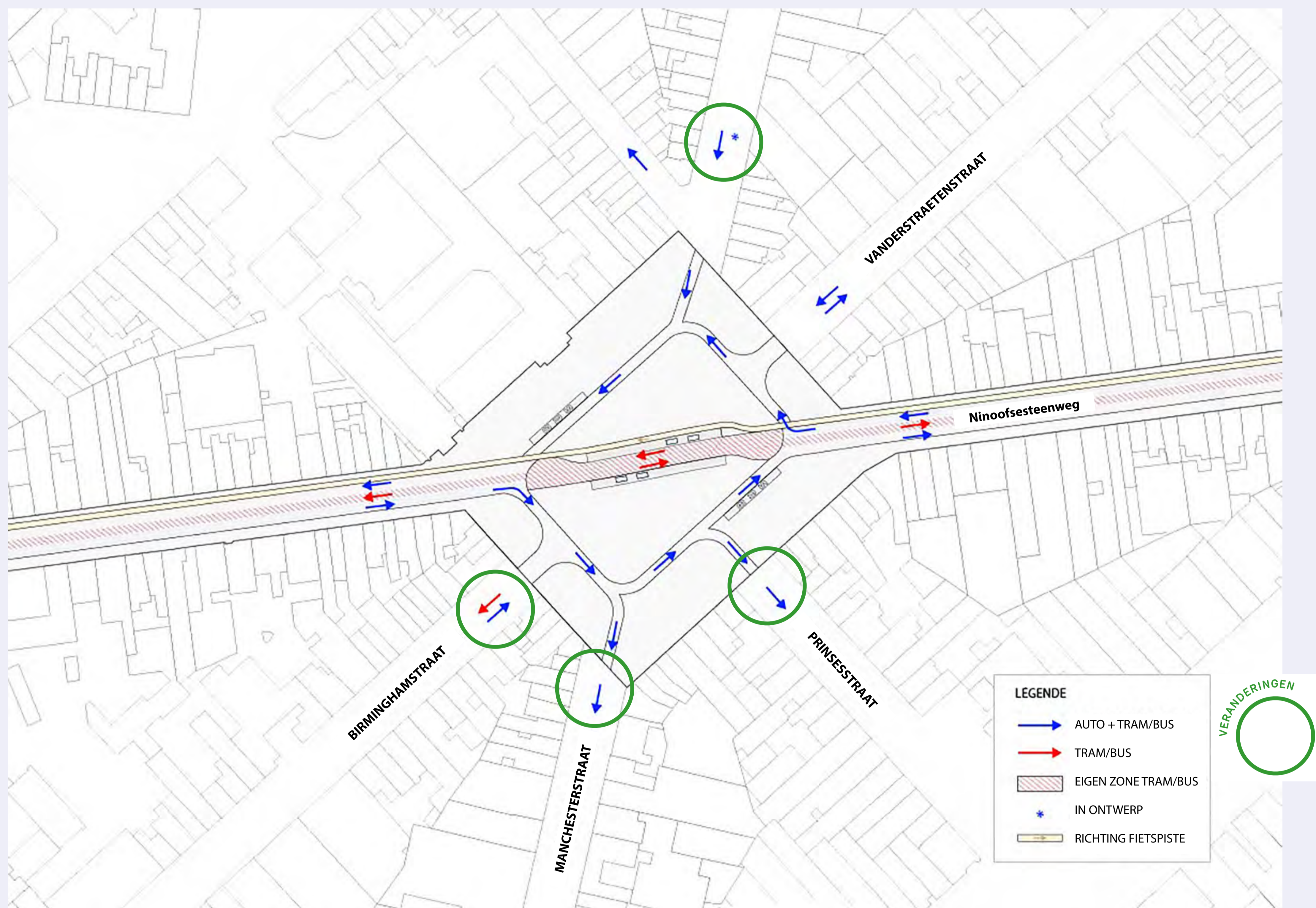
Circulatieplan: ontwerpvoorstel 2
