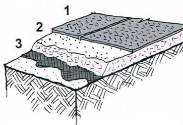
Figure 3: illustration du lit de pose des plaques de répartition de charge : 3 – géotextile, 2 – broyat de branches ou empierrement, 1 – plaques de répartition de charge.
